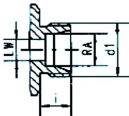
DIN 2353 SR
