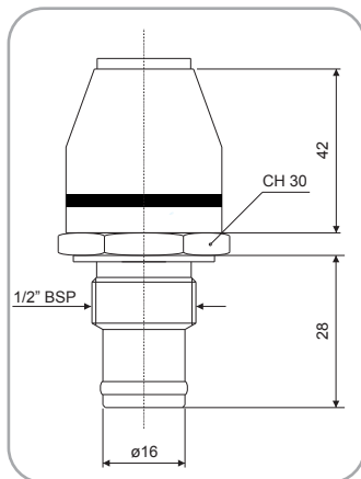
VISUAL INDICATOR
