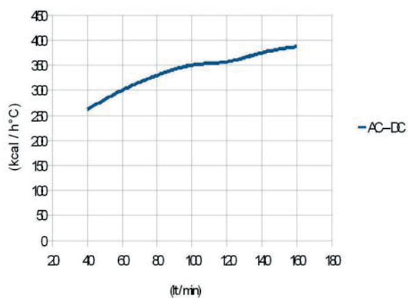
Leistungdiagramm/Performance Diagram
