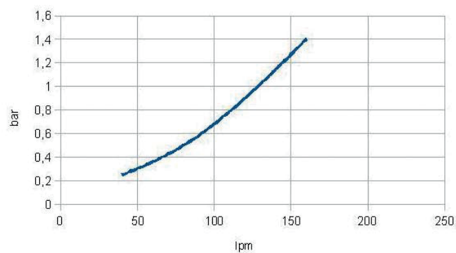
Druckabfall/Pressure Drop
