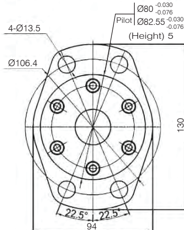
4 Bolt Flange
