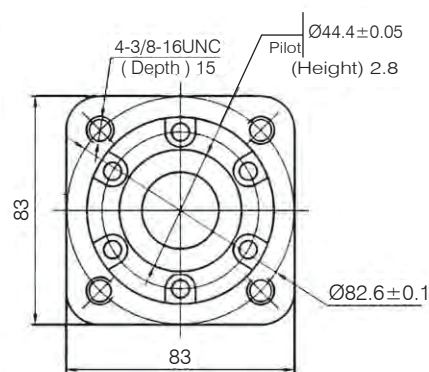
4 Bolt Flange
