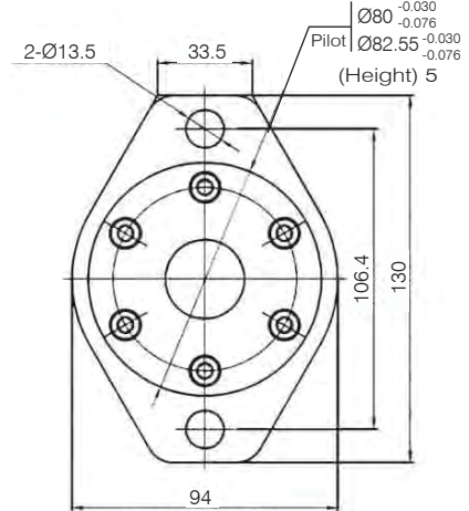
2 Bolt Flange
