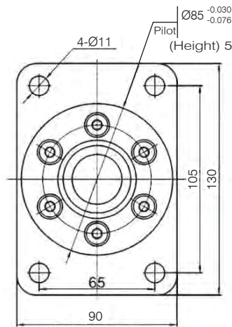
4 Bolt Flange
