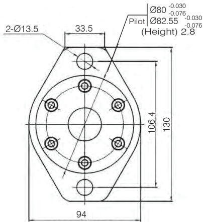
2 Bolt Flange
