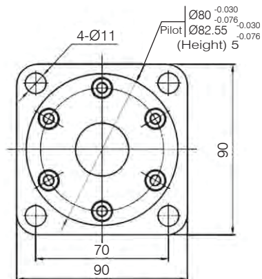
4 Bolt Flange
