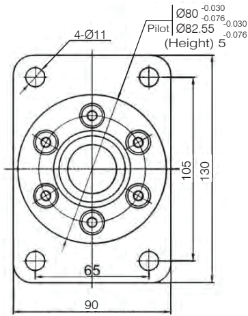
4 Bolt Flange
